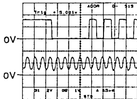
CH1 Y: 2V X: 0.5µs CH2 Y: 1V X: 0.5µs
